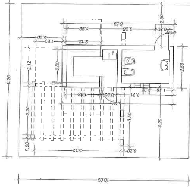
PLANTA COTADA
